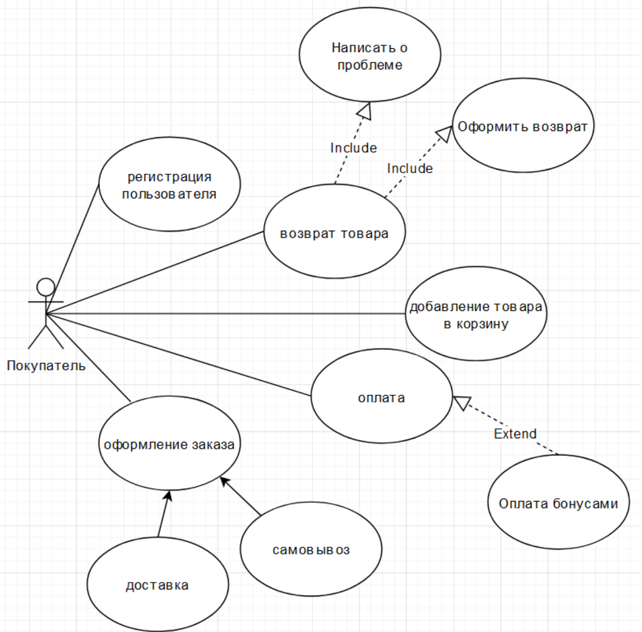
Рисунок 1 – Пример «Диаграммы прецедентов деятельности интернет-магазина»
